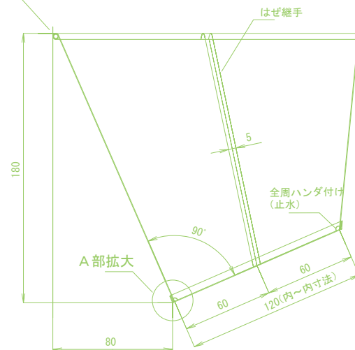
内容器側面詳細
