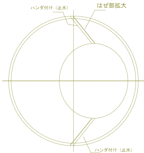
内容器平面詳細 (内部を見る)
