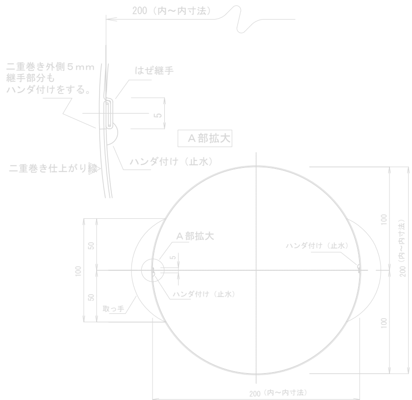
外容器平面詳細 (内部を見る)
